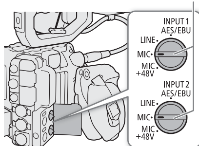
Переключатели INPUT 1/INPUT 2 (выбор источника звука)
